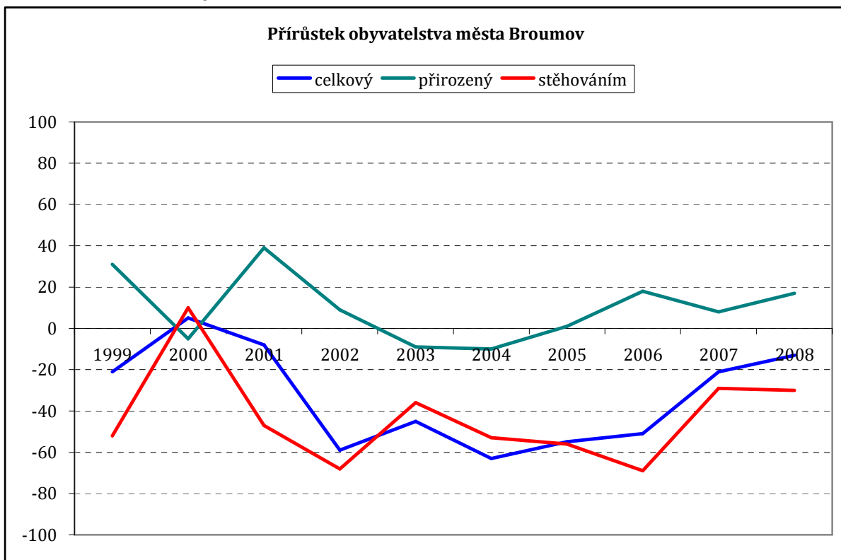
Graf 2: Přírůstek obyvatelstva města Broumov
